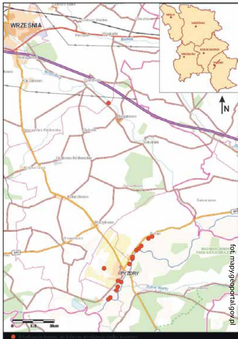
Lokalizacja osuwisk na terenie powiatu wrzesińskiego na tle mapy topograficznej
