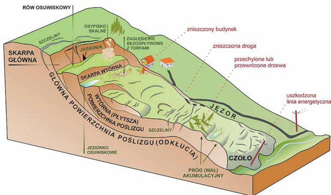
Schemat form osuwiskowych
